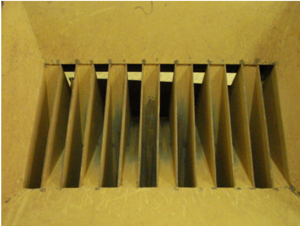
Photo 9 : Echantillonneur à couloires pour préparation échantillons
